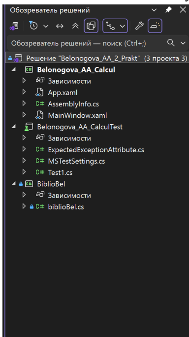
Рисунок 6. Обозреватель
