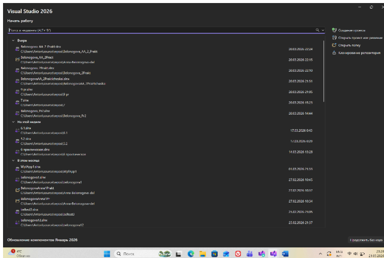
Рисунок 1. Главное окно
