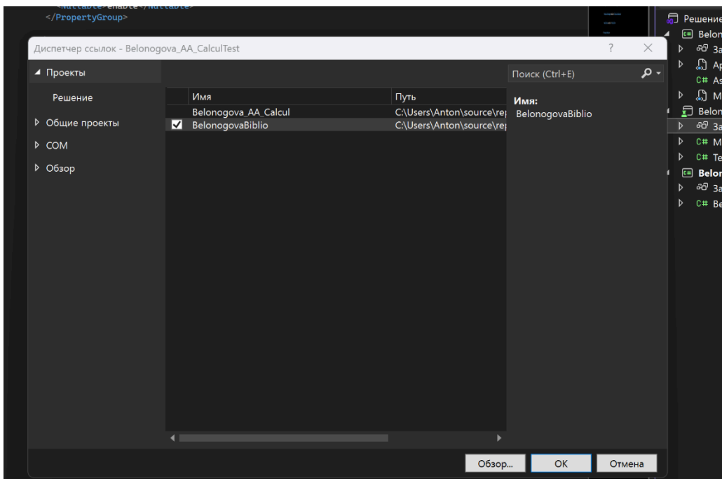
Рисунок 7. Подключение ссылок
