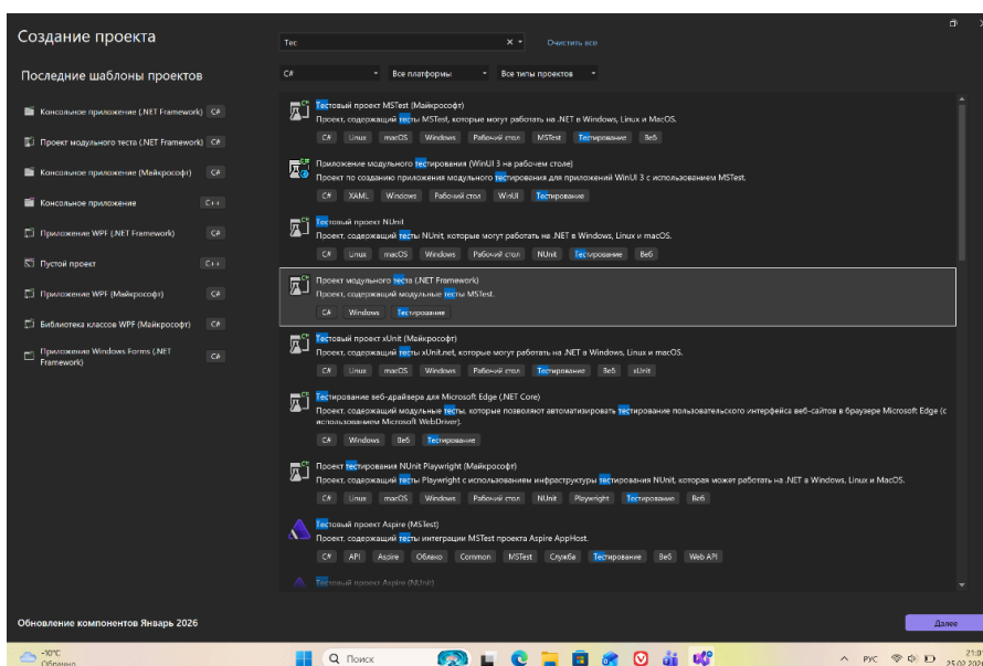
Рисунок 5. Создаем тест
