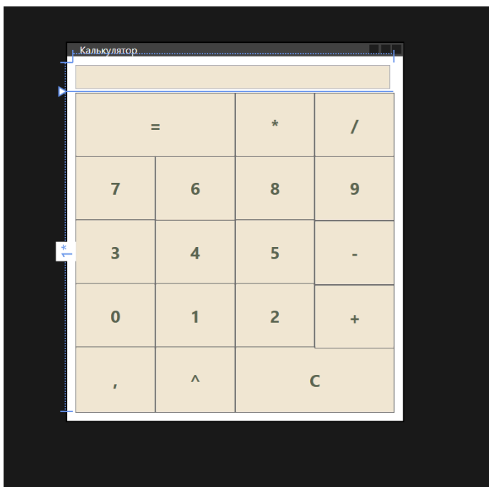
Рисунок 9. Дизайн калькулятора
